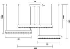
Габаритные размеры
